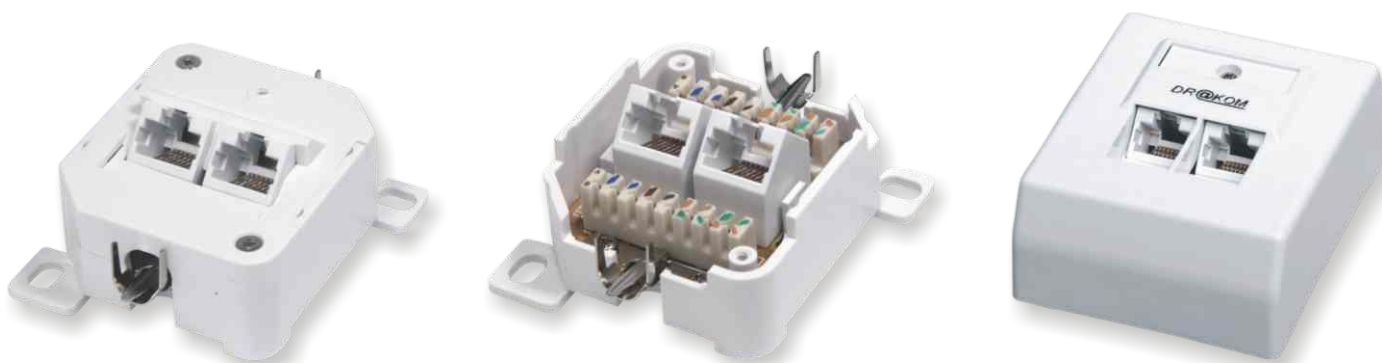
Gniazdo DR@KOM, 2 x RJ45, nieekranowane, Kat. 6, natynkowe
