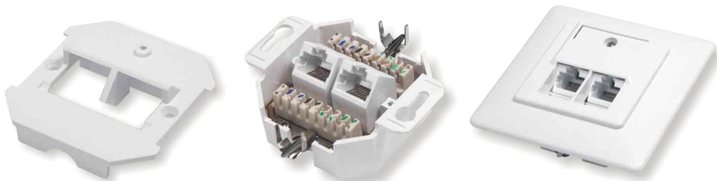
Gniazdo DR@KOM, 2 x RJ45, nieekranowane, kat. 6, podtynkowe
